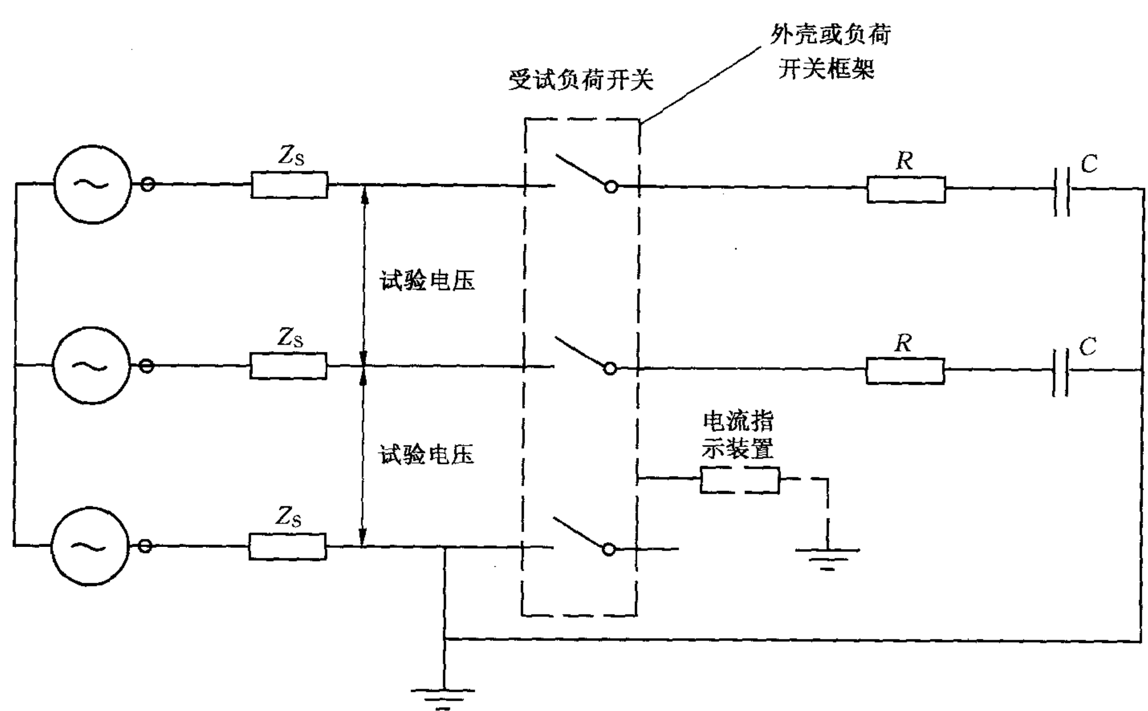
图 9 接地故障条件下电缆充电开断电流试验(试验方式 6b)的三相试验回路
