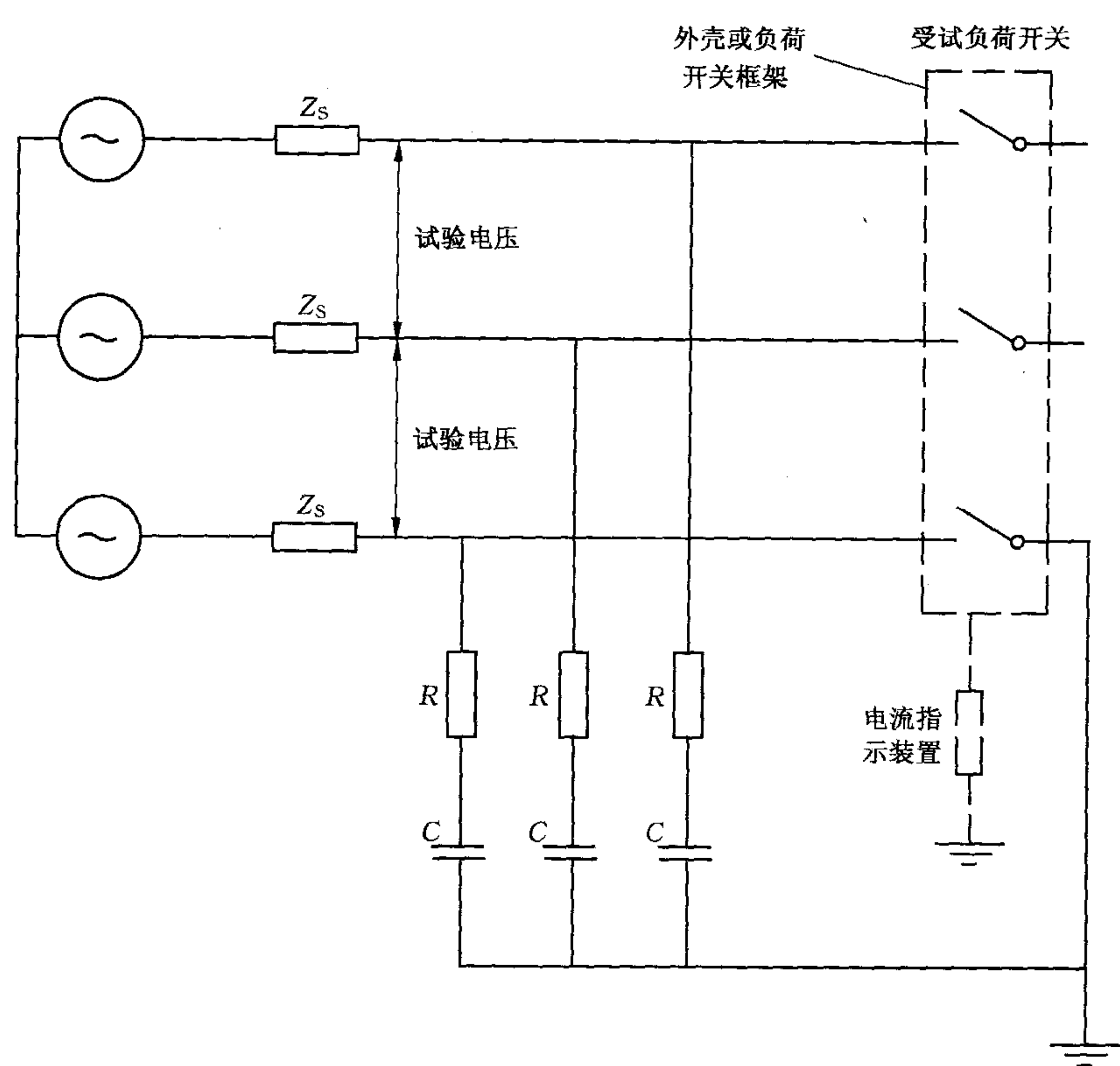
图 8 接地故障开断电流试验(试验方式 6a)的三相试验回路
