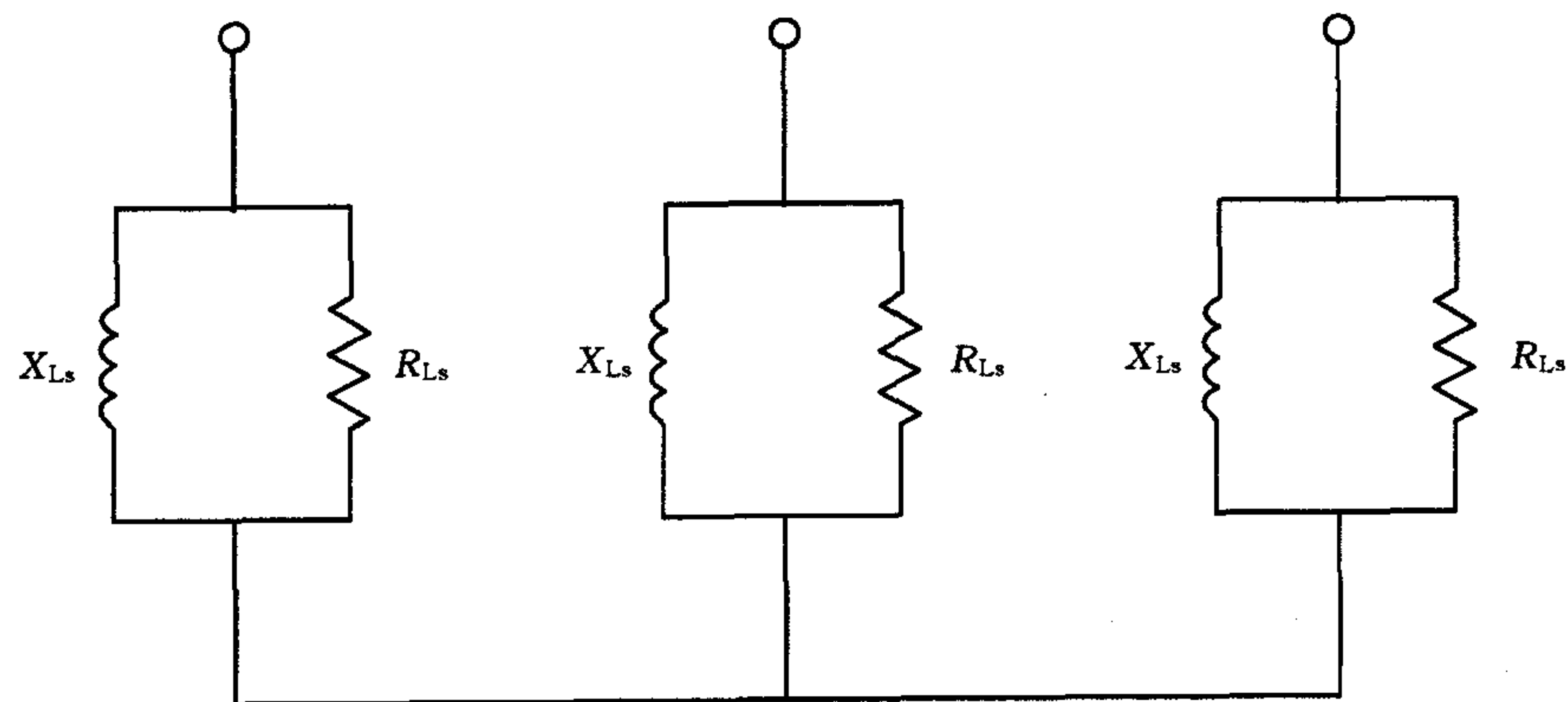
图 1c 星形连接的负载
