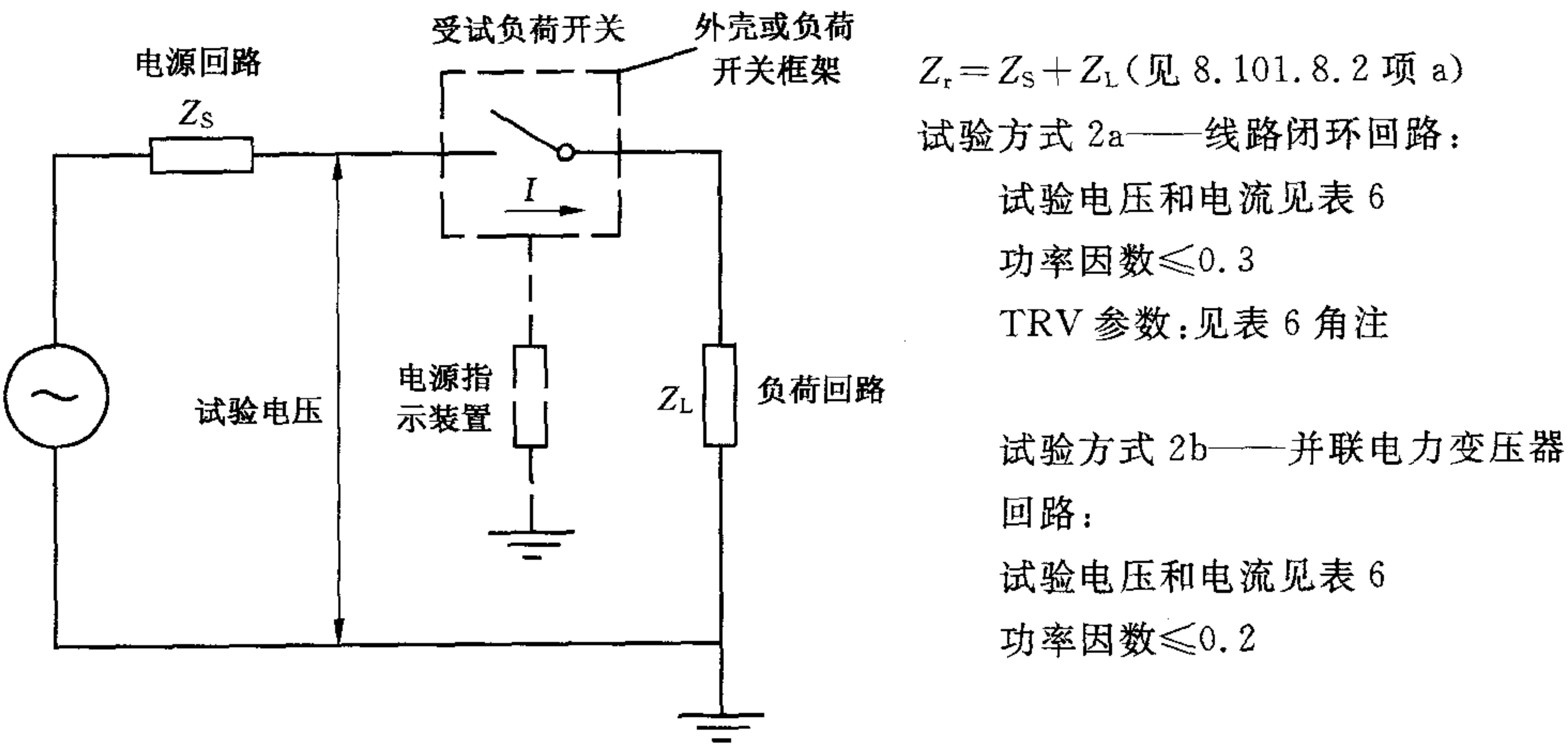
图 4 配电线路闭环和并联变压器闭环电流开合试验(试验方式 2a 和 2b)的单相试验回路
